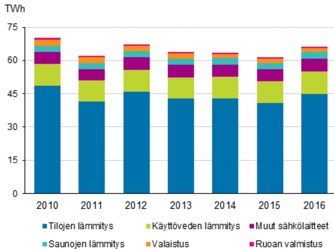
Asumisen energiankulutus 2010-2016
